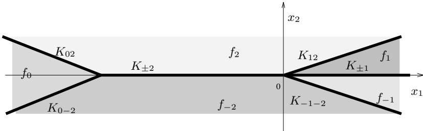
Fig. 9.2. Minimax function
