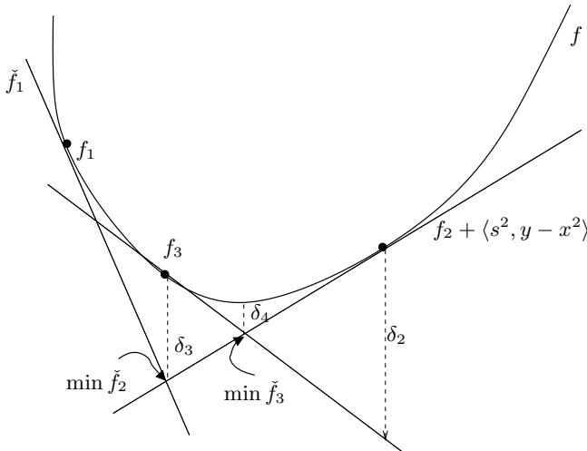
Fig. 9.7. Cutting-planes iterations
