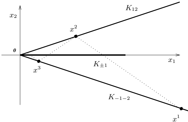
Fig. 9.3. Zigzagging trajectory
